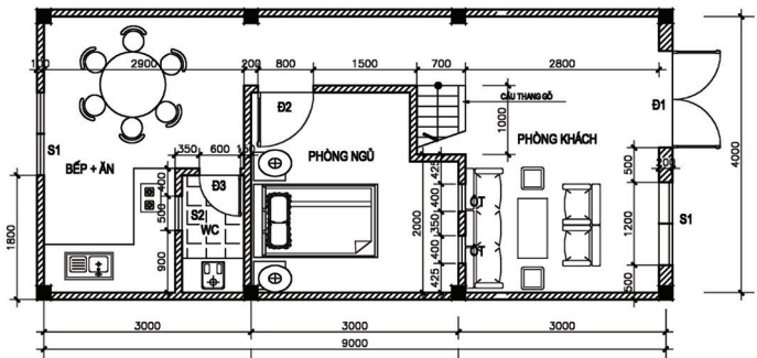
MẶT BẰNG
