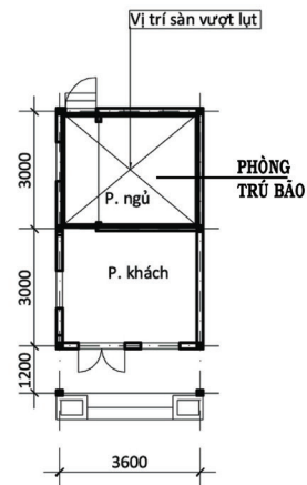
MẶT BẰNG
