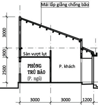
MẶT CẮT
