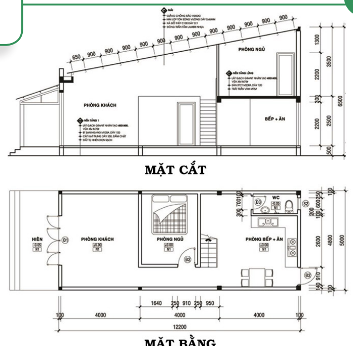
MẶT BẰNG
