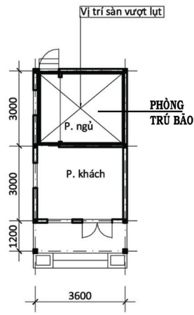
MẶT BẰNG
