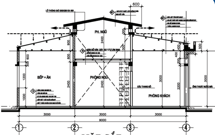
MẶT CẮT
